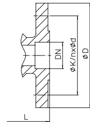
Fig. 634....1 com flanges
