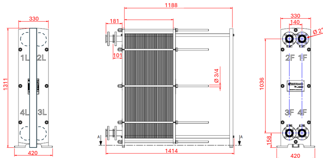
Canais standard – com pontos de contato. Canais médios: 1,80 [mm]
