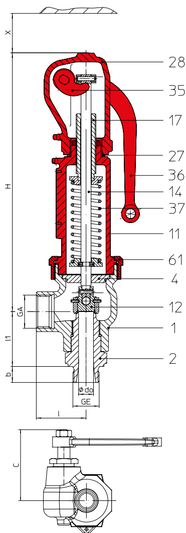
Fig. ... 941 Capuz fechado com alavanca, castelo fechado
