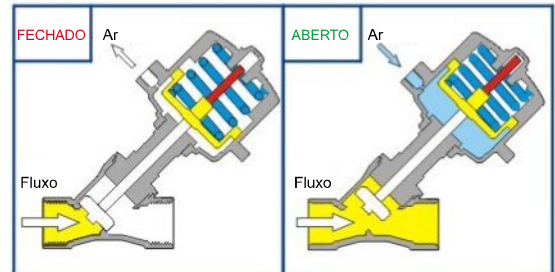
Fechamento contra o sentido do fluxo
