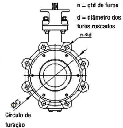
121L Corpo tipo lug
