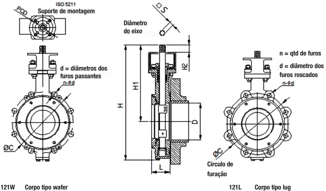
121W Corpo tipo wafer
