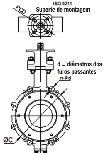
121W Corpo tipo wafer
